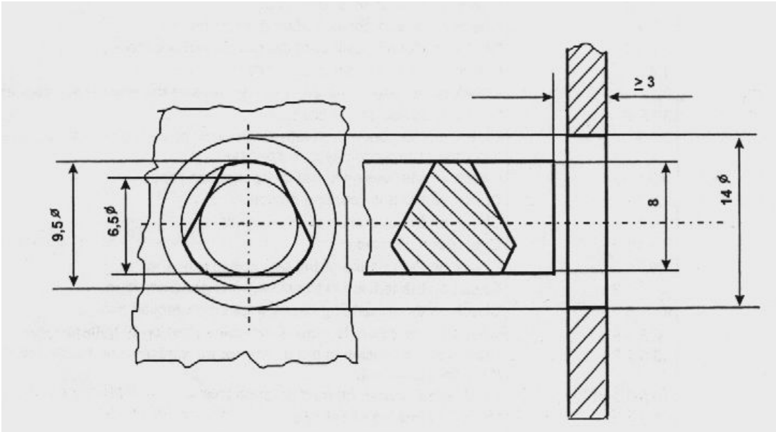
شکل ب- ۱: کلید سه گوش
