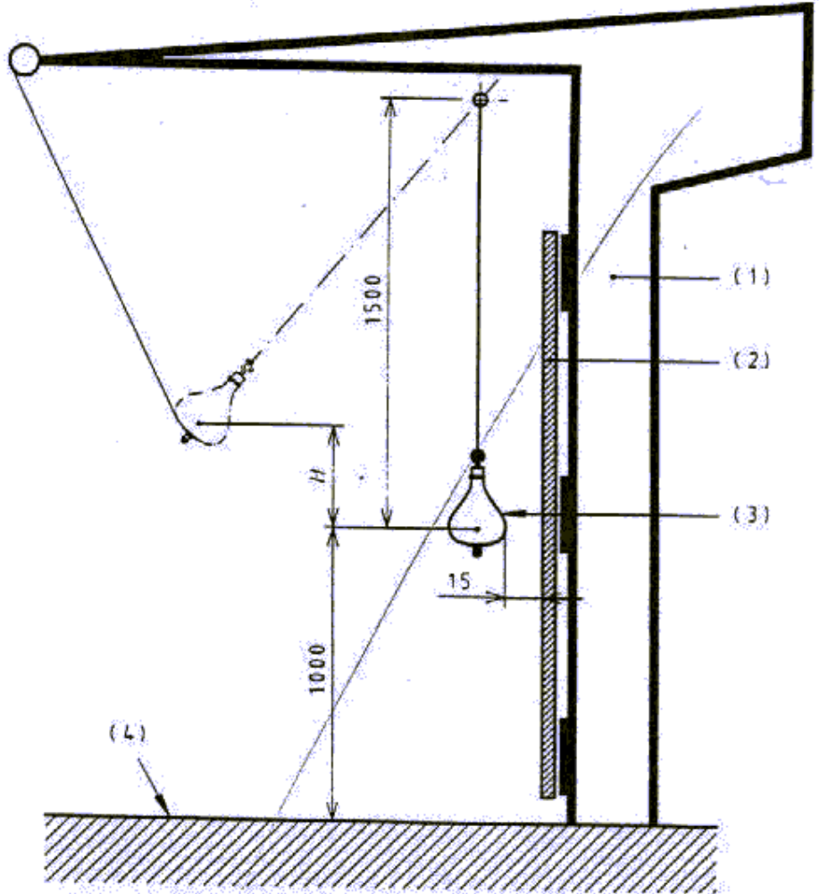
شکل خ- ۲ : وسیله ضربه آونگی نرم
