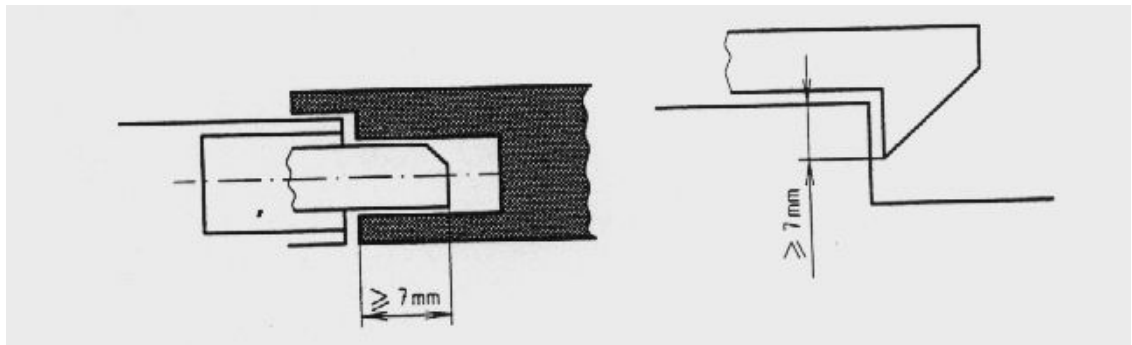
شکل ۳: مثالهایی از اجزاء قفل کننده
